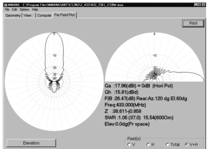
Joonis 3: ES0W ANTENNA CHARACTERISTICS MMANA (Z = 38 ohm)
